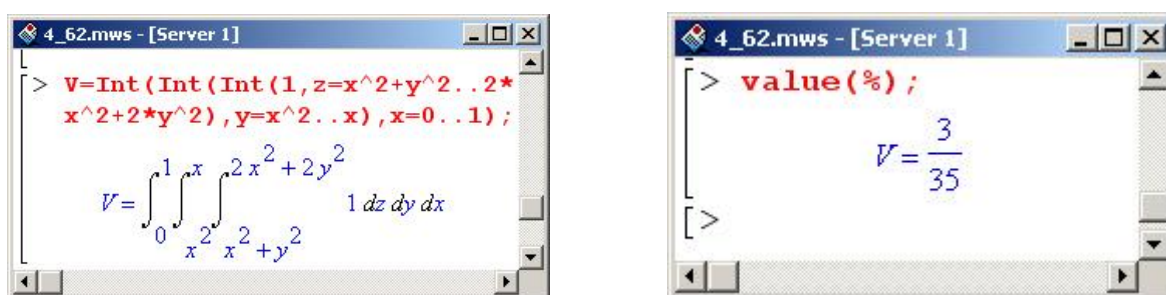
а) б) Рис. 3. Визначення меж інтегрування
