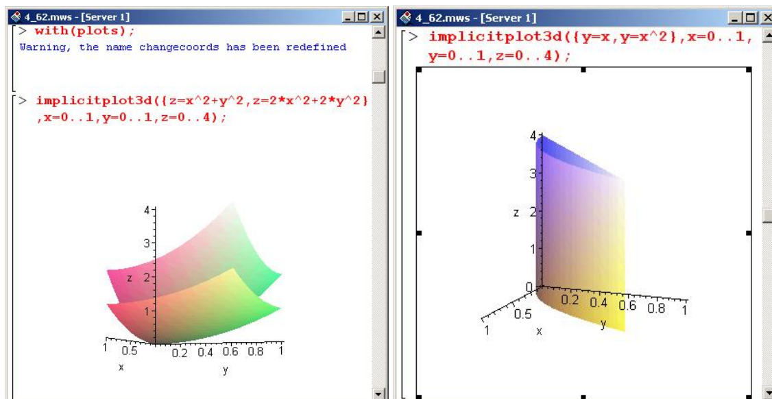
а) б) Рис. 2. Наочне подання області інтегрування
