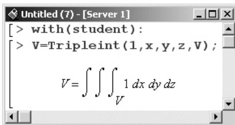
Рис. 1. Обчислення потрібного інтегралу
