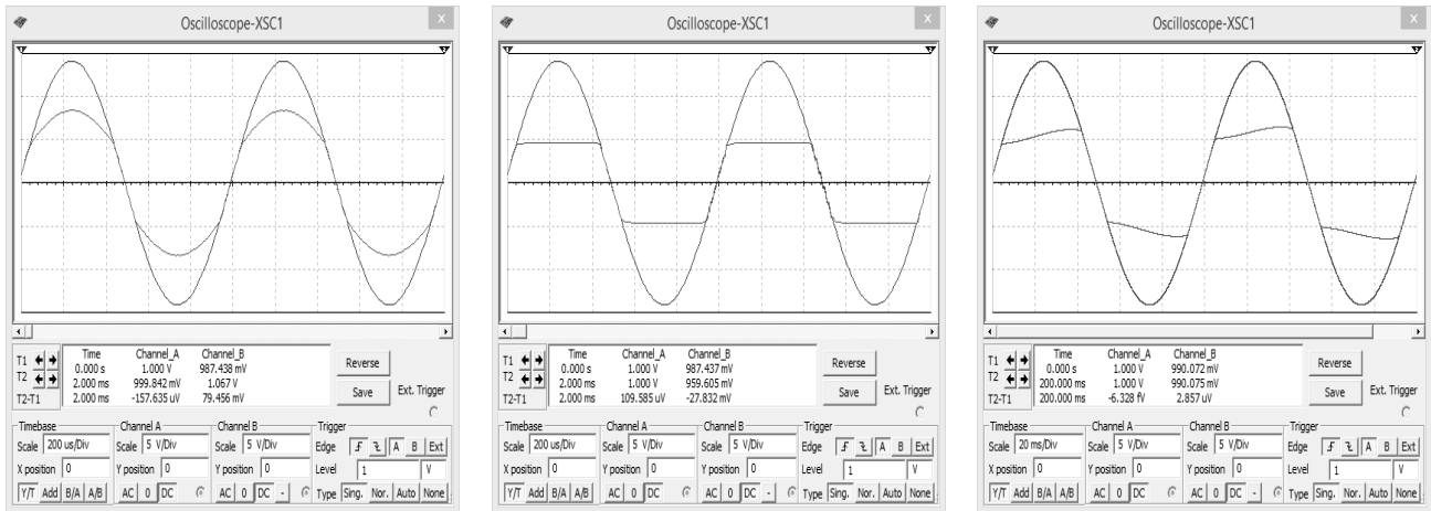
Рис. 4. Осцилограми сигналів на виході обмежувача за відсутності конденсаторів (а), при наявності конденсаторів на частоті сигналу 1000 Гц (б) та частоті сигналу 10 Гц (в)
